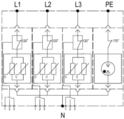
Принципиальная схема
