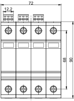
Габаритные размеры
